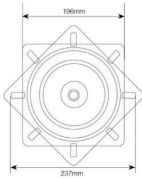
材质厚度: 2.0mm/2.5mm 尺寸:200x200mm转盘
