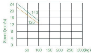
速度与负载关系图 Speed vs load
