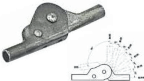
C-216-8带孔正五档180° 日本扣
