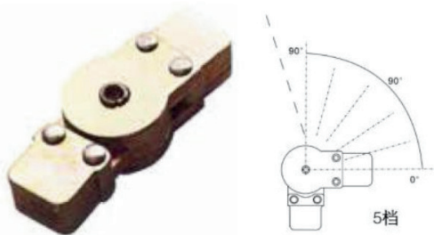
C-26-2C反五档千层铰
