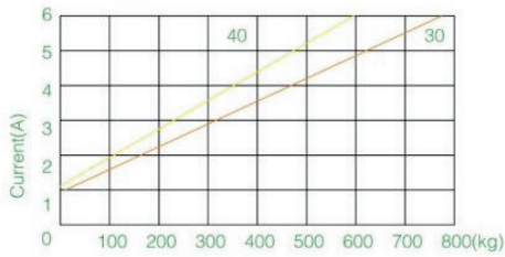
C-803电动推杆
