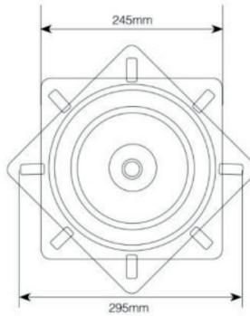
材质厚度 2.0mm/2.5mm/3.0mm 尺寸/Size:250x250mm转盘
