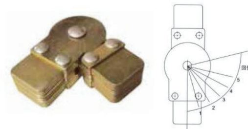
C-26H 正五档千层铰
