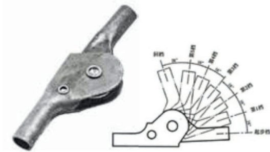
C-28-1正五档90° 大日本扣 Big wheel hinge
