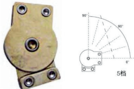
C-26-2B短边反五档千层铰
