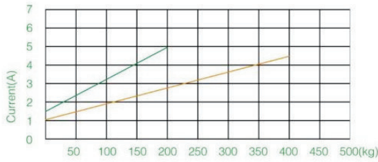
电流与负载关系图 Current vs load
