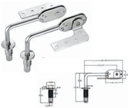
C-6A-7头枕铰链
