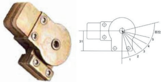
C-26-2A反五档千层铰
