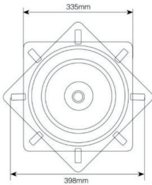
材质厚度: 2.5/3.0mm 尺寸/Size:330x330mm转盘
