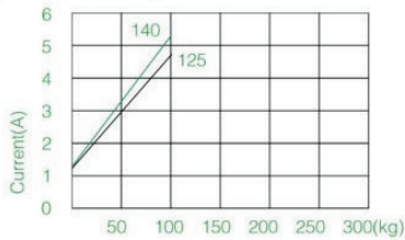
电流与负载关系图 Current vs load
