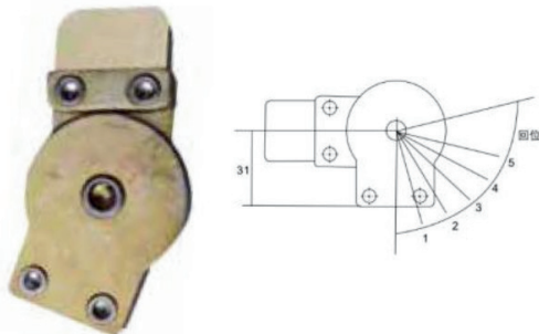
C-26-2D反五档千层铰
