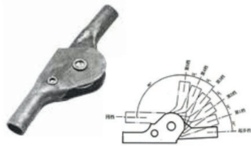
C-28-2正五档180° 大日本扣 Big wheel hinge
