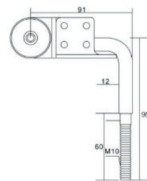
C-338D 单耳头枕
