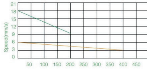
速度与负载关系图 Speed vs load
