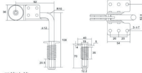
C-338E 双耳头枕 三档/六档
